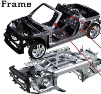
図19 D-FRAME
