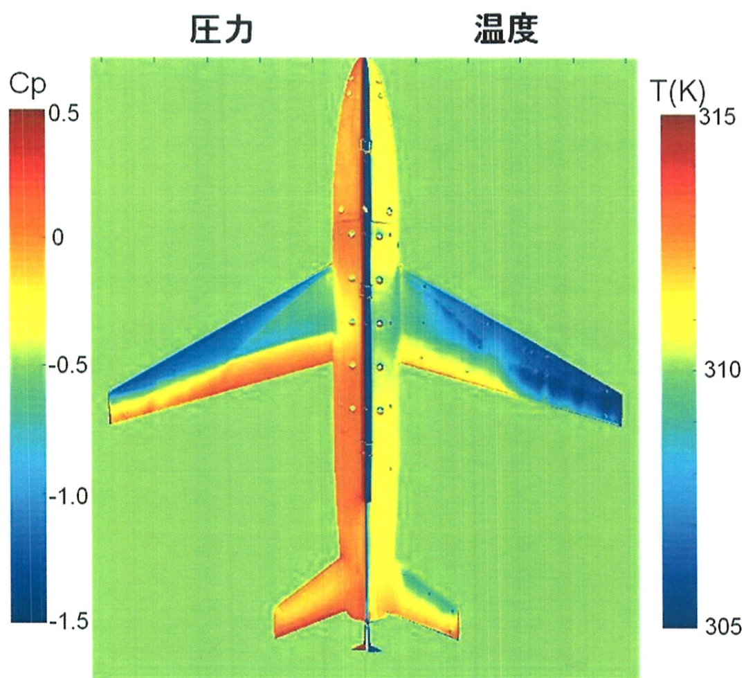
図 1 感圧／感温塗料計測結果の例 (マッハ数=0.78、迎角=0°、総圧=100kPa) (Vol.48 No. 3 p104 に掲載)
